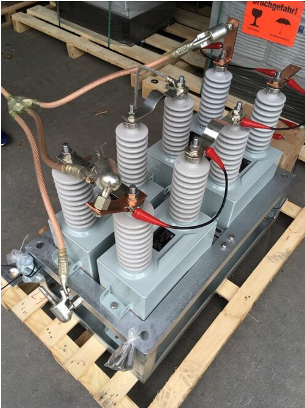
Beispiel einer kurzgeschlossenen, geerdeten, in Reihe geschalteten Kondensatorbank. Ohne allpoliges Erden und Kurzschließen mithilfe eines Erdungs- und Kurzschliessseils, ist das Arbeiten daran nicht zulässig. (Quelle: Condensator Dominit)
