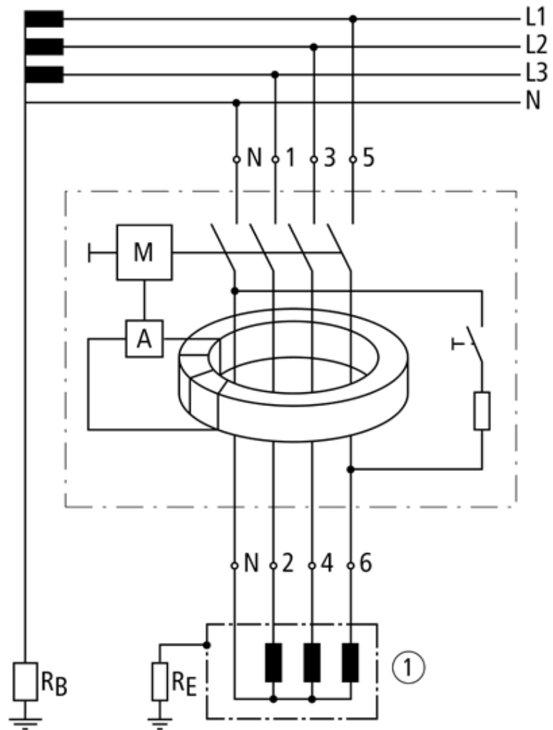
Abb. 2: Prinzipieller Aufbau eines Fehlerstrom-Schutzschalters mit netzspannungsunabhängiger Auslösung nach DIN EN 61008-1 (VDE 0664-10)
