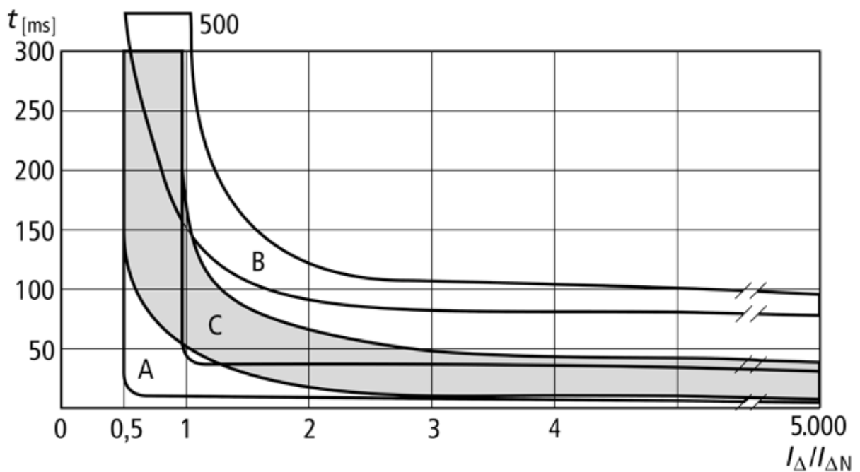
Abb. 6: Auslösekennlinien von unverzügerten (A), verzögerten, selektiven (B) und kurzzeitverzögerten (C) Fehlerstrom-Schutzschaltern
