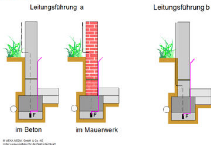
Abb. 1: Fundamenteerder: Verlegung und Leitungsführung (Bildquelle: Unterweisungsfolien für die Elektrofachkraft)
