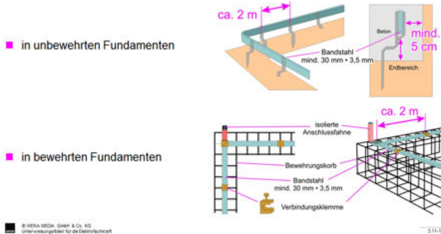
Abb. 2: Anordnung des Fundamenterders (Bildquelle: Unterweisungsfilme für die Elektrofachkraft)
