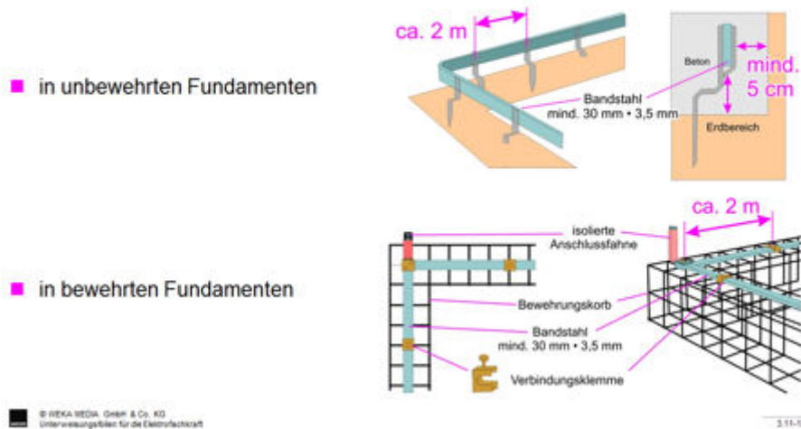
Abb. 2: Anordnung des Fundamenterders (Bildquelle: Unterweisungsfolien für die Elektrofachkraft)
