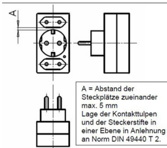
Konformer Adapter mit Schutzkontaktsteckplatz
