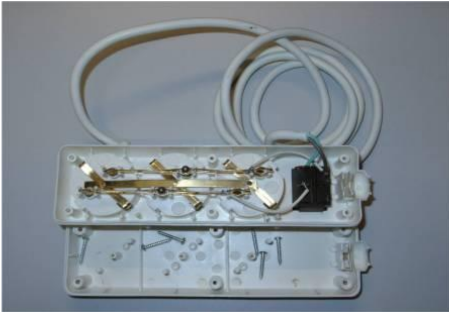
Abb. 3: Geöffnete Steckdosenleiste
